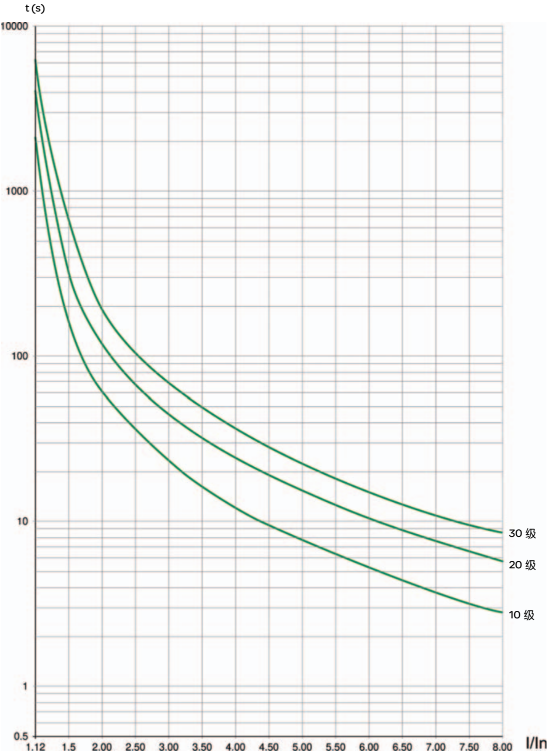
热态曲线
